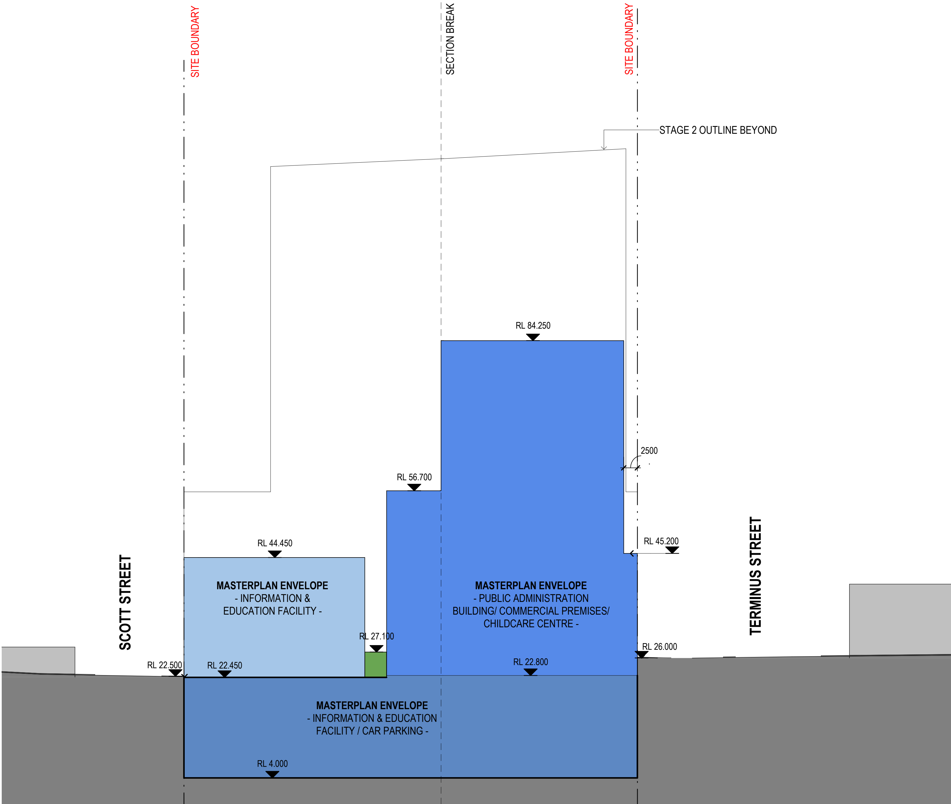
1 SECTION B 1 : 400
