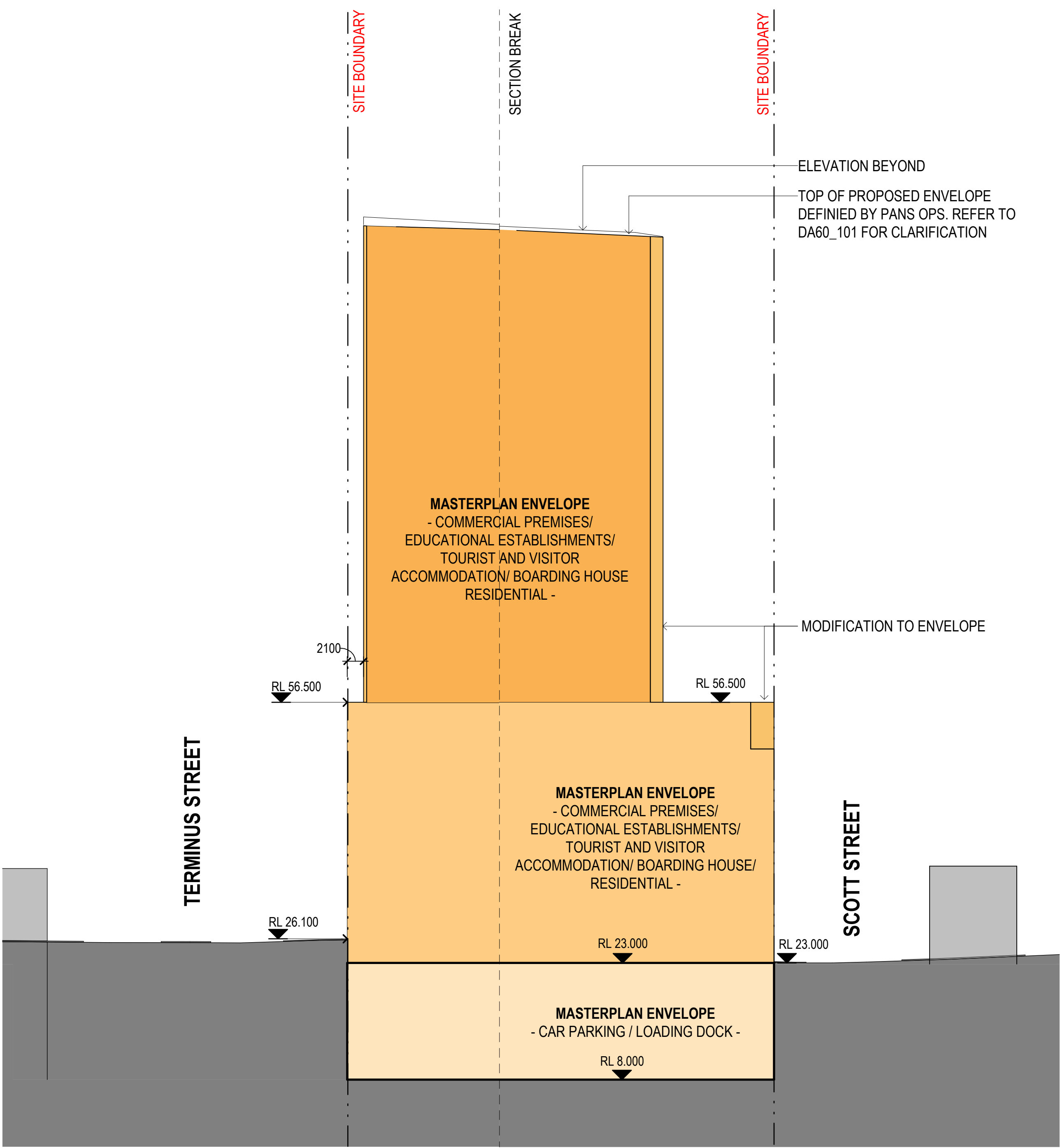
2 SECTION C 1 : 400
