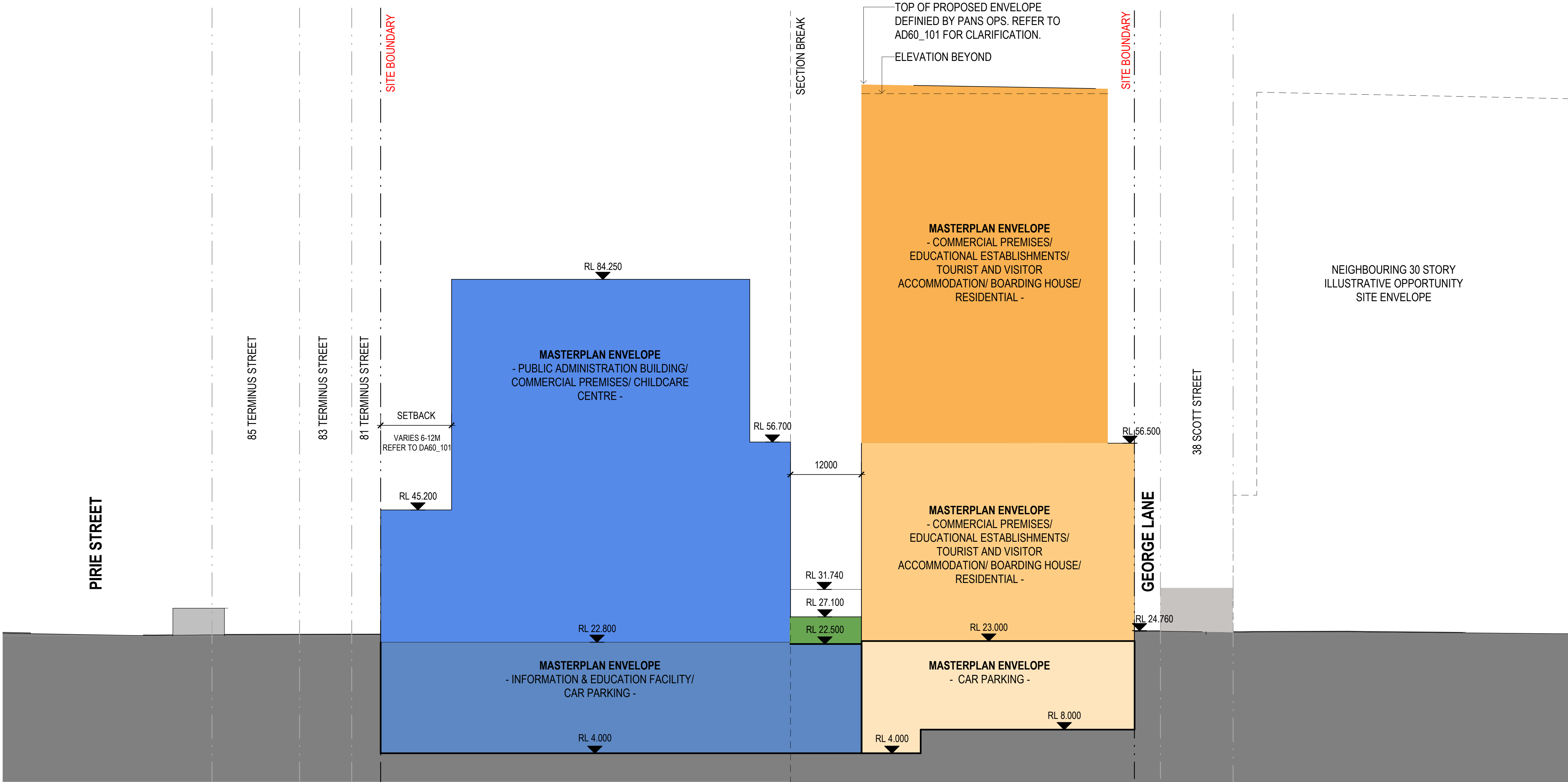
1 SECTION A 1 : 400
